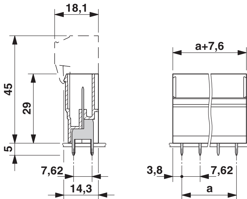
Rysunek wymiarowy
