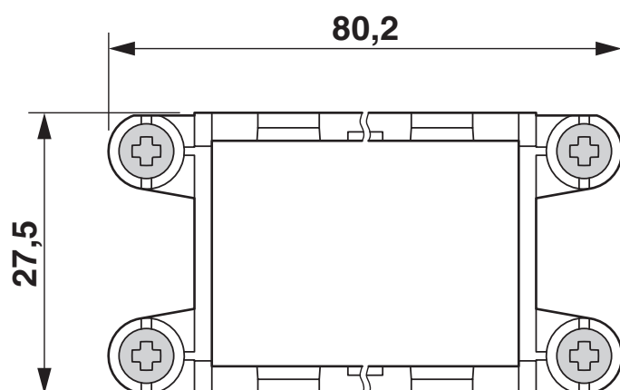
Rysunek wymiarowy
