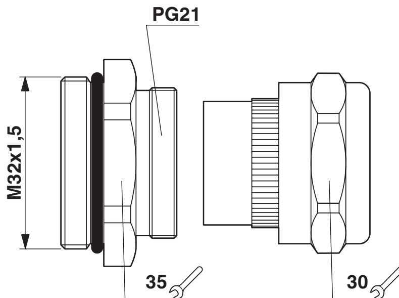
Rysunek wymiarowy
