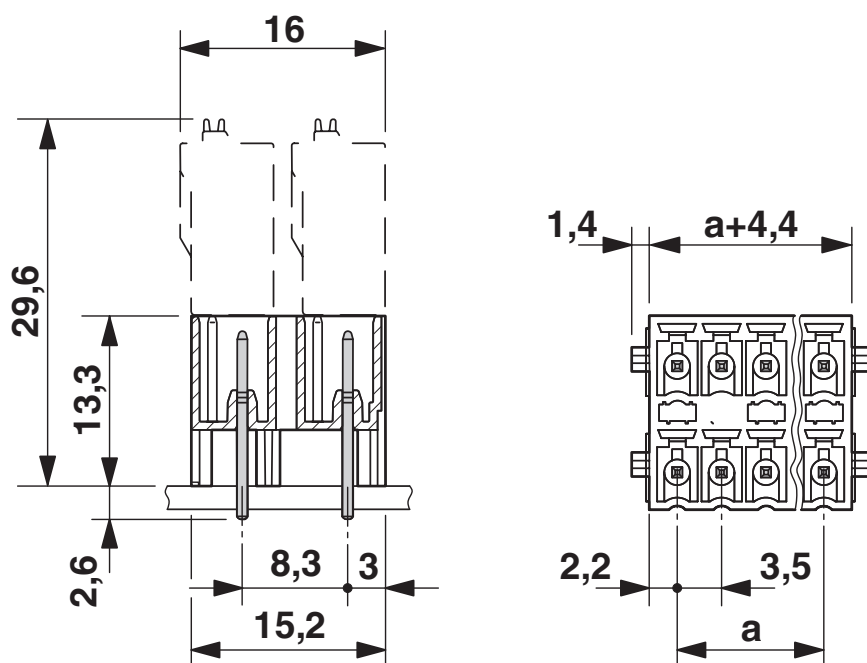
Rysunek wymiarowy
