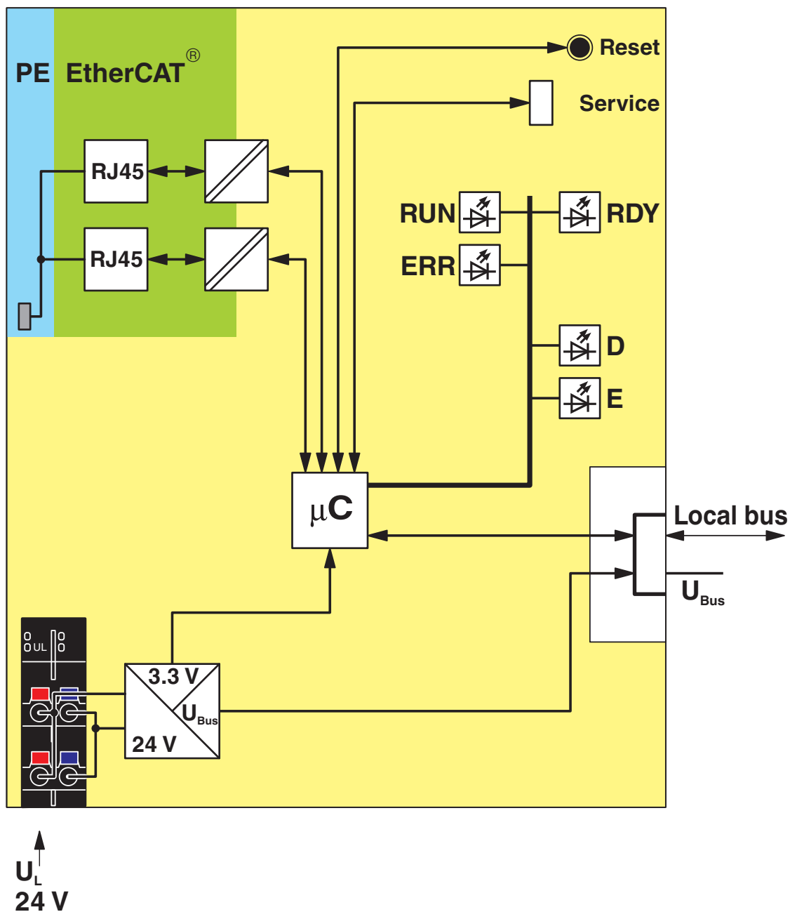
Schemat blokowy
