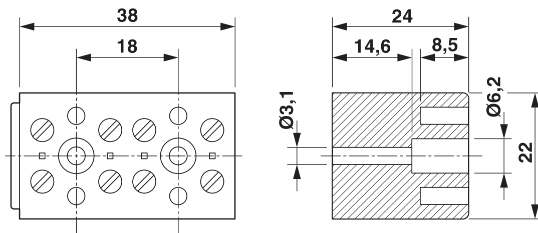
Rysunek wymiarowy
