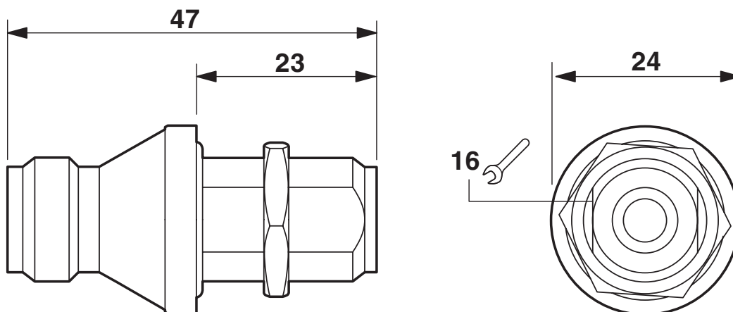
Rysunek wymiarowy
