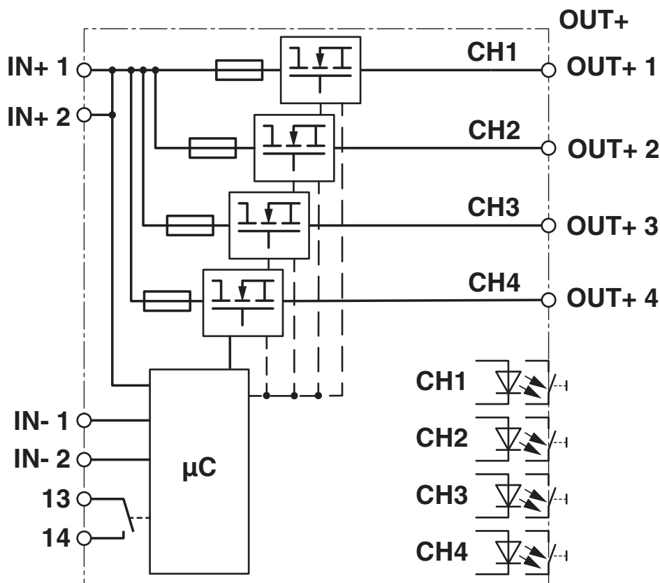
Schemat blokowy
