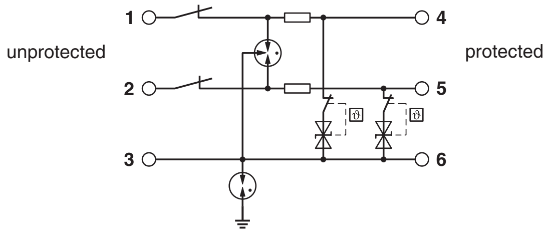
Schemat
