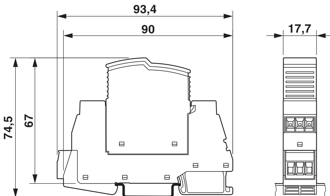
Rysunek wymiarowy
