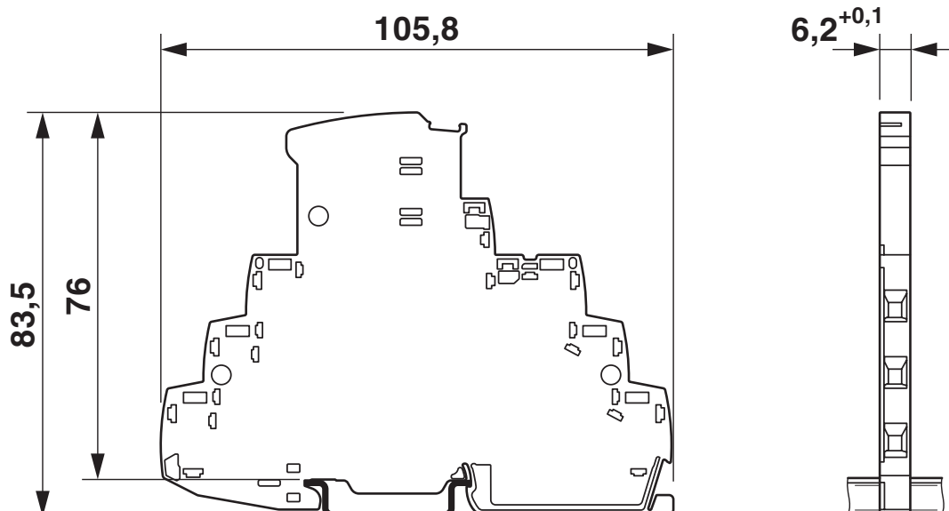
Rysunek wymiarowy
