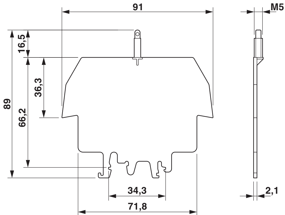
Rysunek wymiarowy
