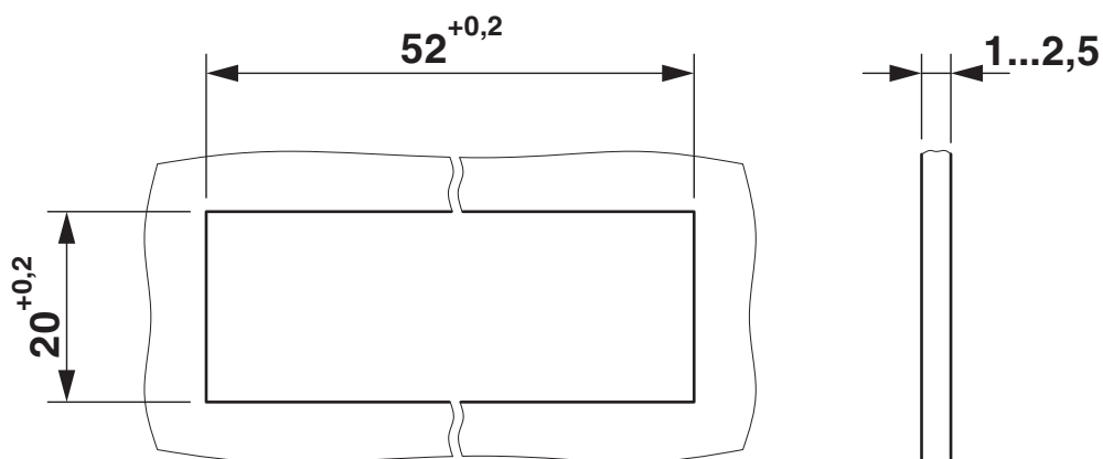
Rysunek wymiarowy
