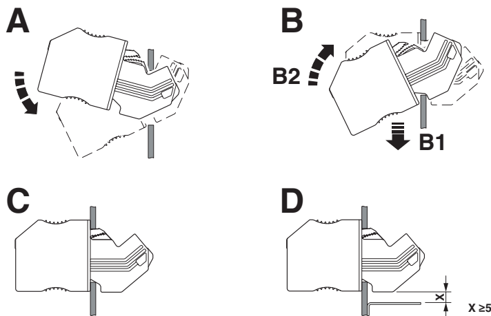
Rysunek schematyczny
