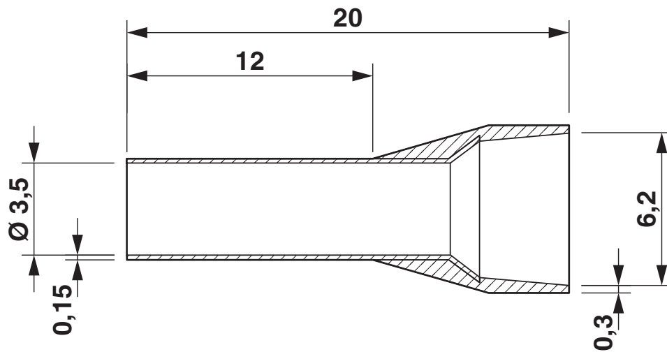
Rysunek wymiarowy
