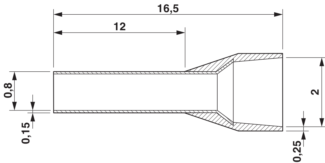
Rysunek wymiarowy
