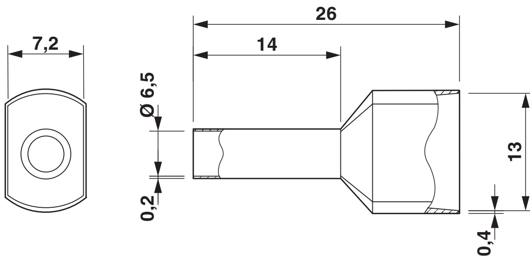
Rysunek wymiarowy
