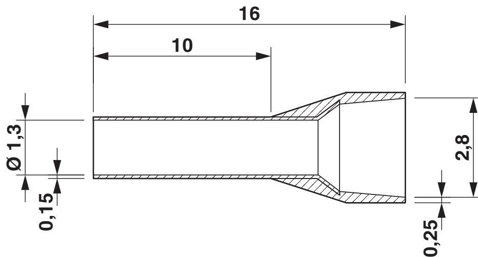
Rysunek wymiarowy
