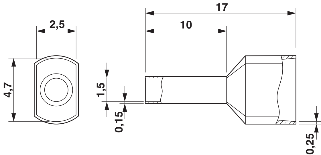
Rysunek wymiarowy
