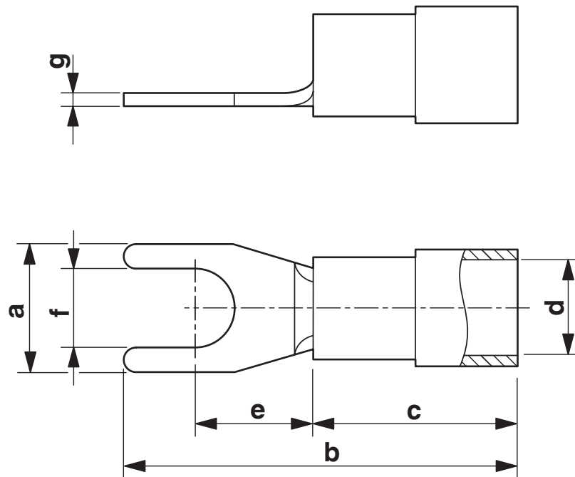
Rysunek wymiarowy
