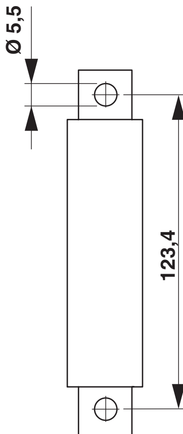
Rysunek wymiarowy
