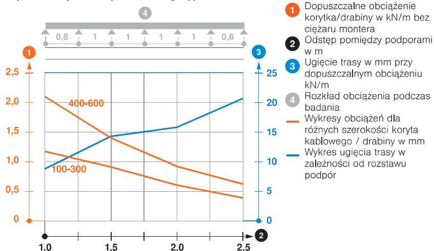
Wykres obciążenia korytka kablowego typu RKSM 60
