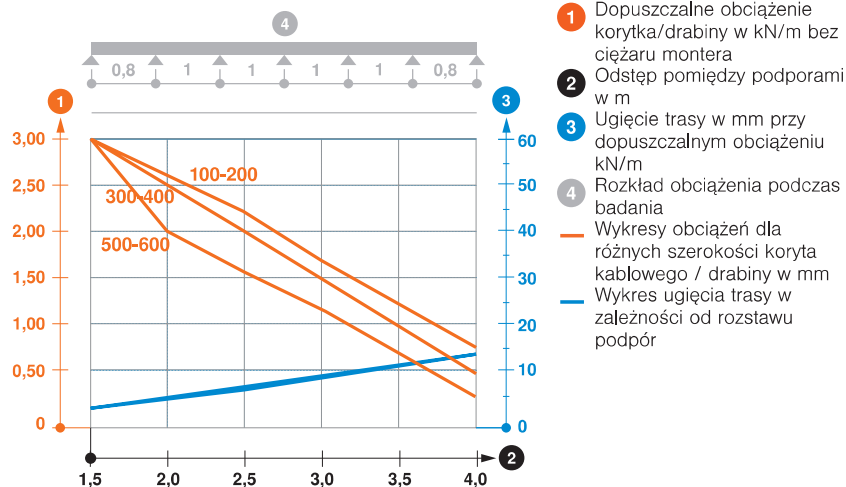
Wykres obciążenia koryta kablowego typ SKSM 110
