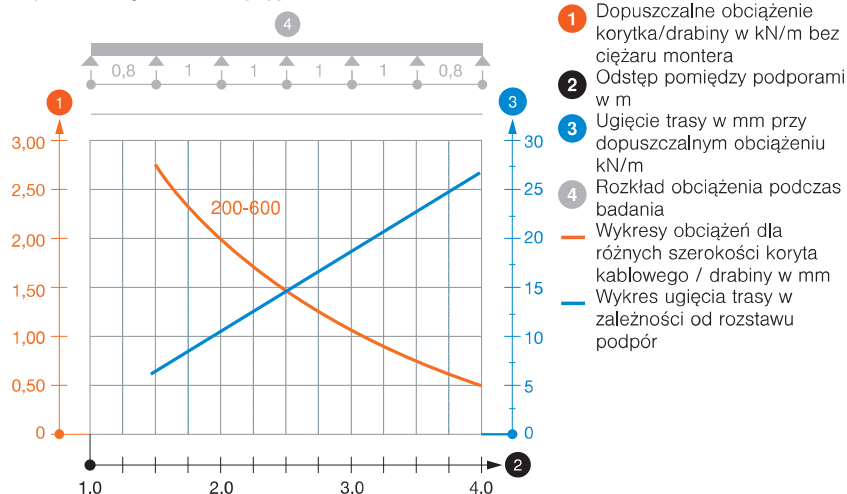
Wykres obciążenia drabiny typ SLG 45 NS
