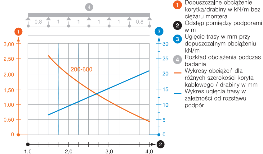
Wykres obciążenia LG 60 NS
