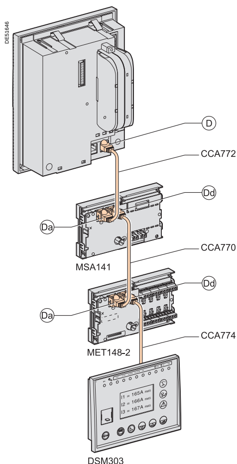
Exemple de chaînage des modules pour Sepam série 20.
