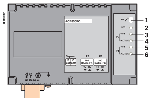
ACE850FO : vue de face.
