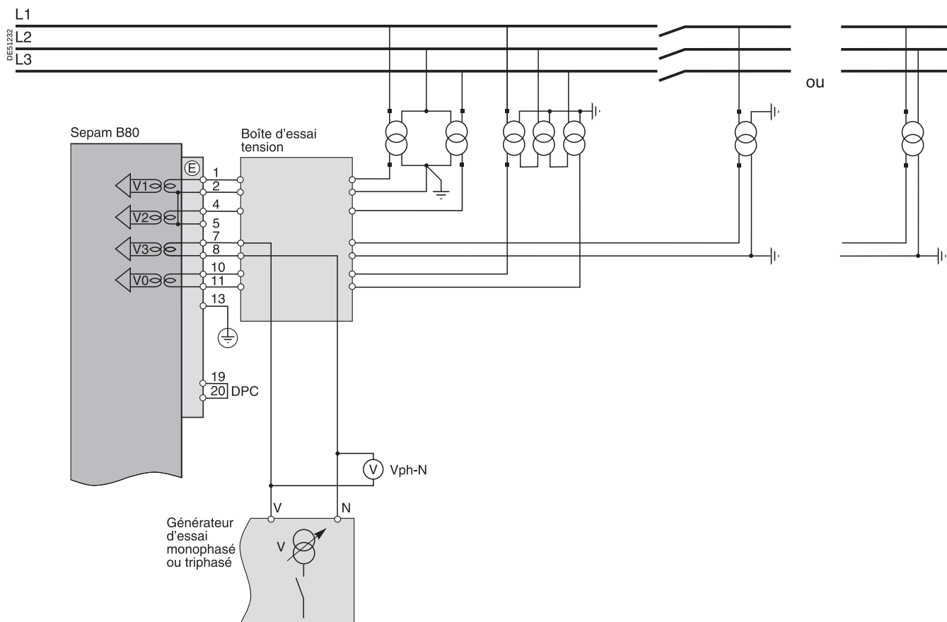
Schéma de principe n° 2
