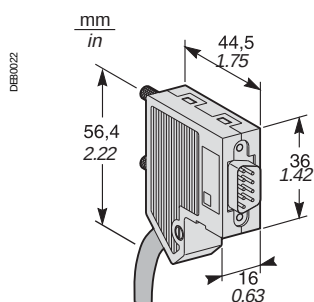
Connecteur sub-D 9 broches mâle livré avec l'ACE919.
