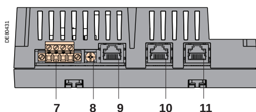
ACE850TP : vue de dessous.
