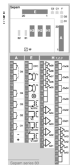
Etiquette d'identification des borniers.
