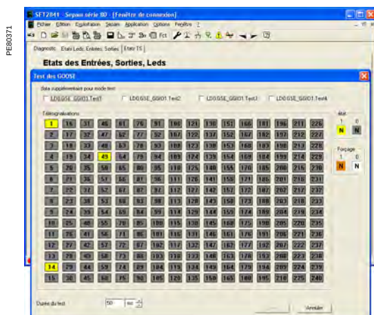
SFT2841 : test des entrées logiques GOOSE.
