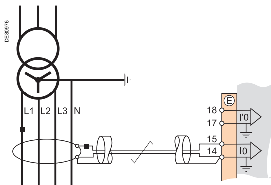
Raccordement sur réseaux TN-S et TT.
