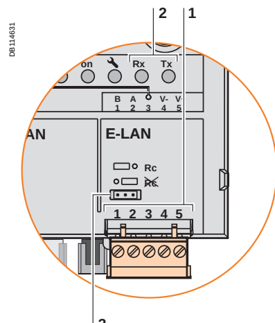
Port E-LAN (ACE969TP-2 ou ACE969FO-2)
