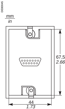
Vue avant capot levé.
