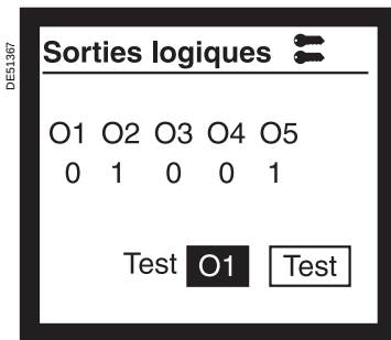
Écran de présentation des sorties logiques de l'unité de base, avec l'état de chaque sortie et la possibilité de tester chaque sortie.
