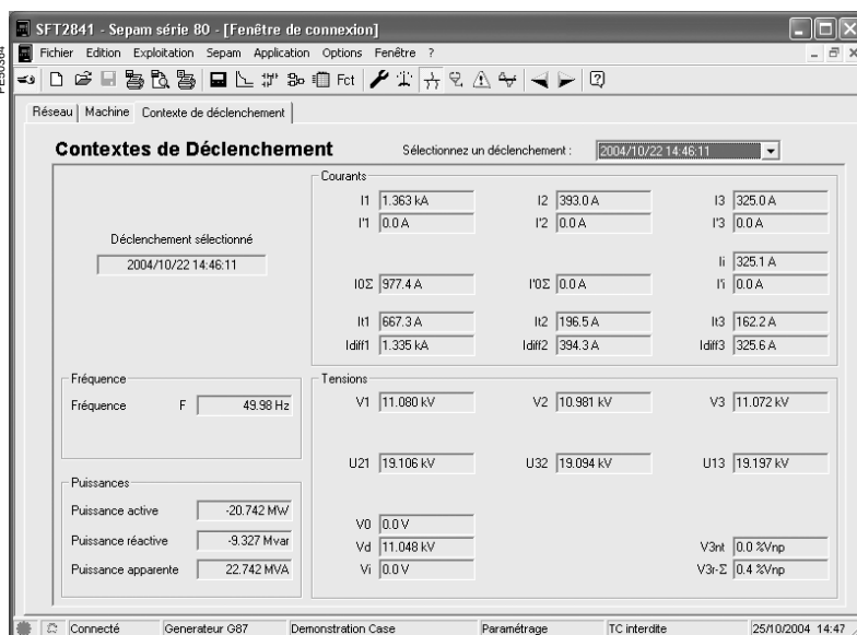
Exemple d'écran de contextes de déclenchement.
