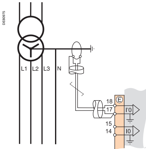
Raccordement sur réseau TT.
