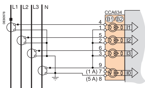
Raccordement sur réseaux TN-S et TT.
