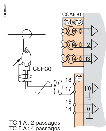
Raccordement avec CSH30.
