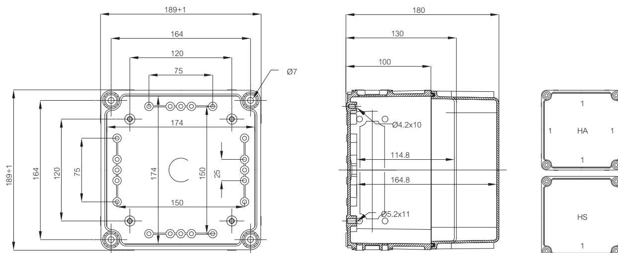
EK 190x190x130-180
