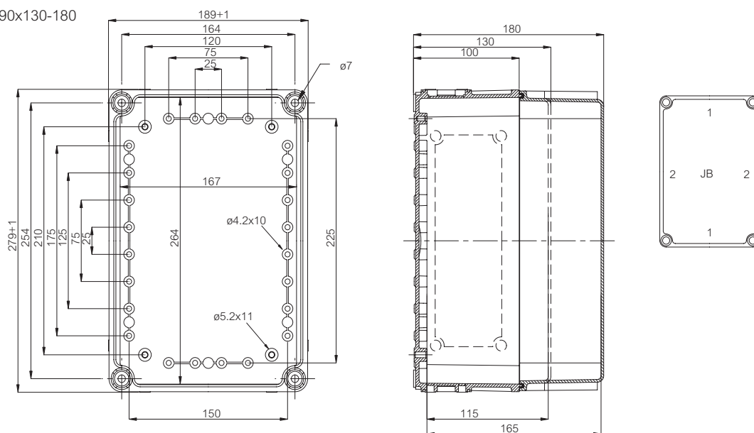
EK 280x190x130-180
