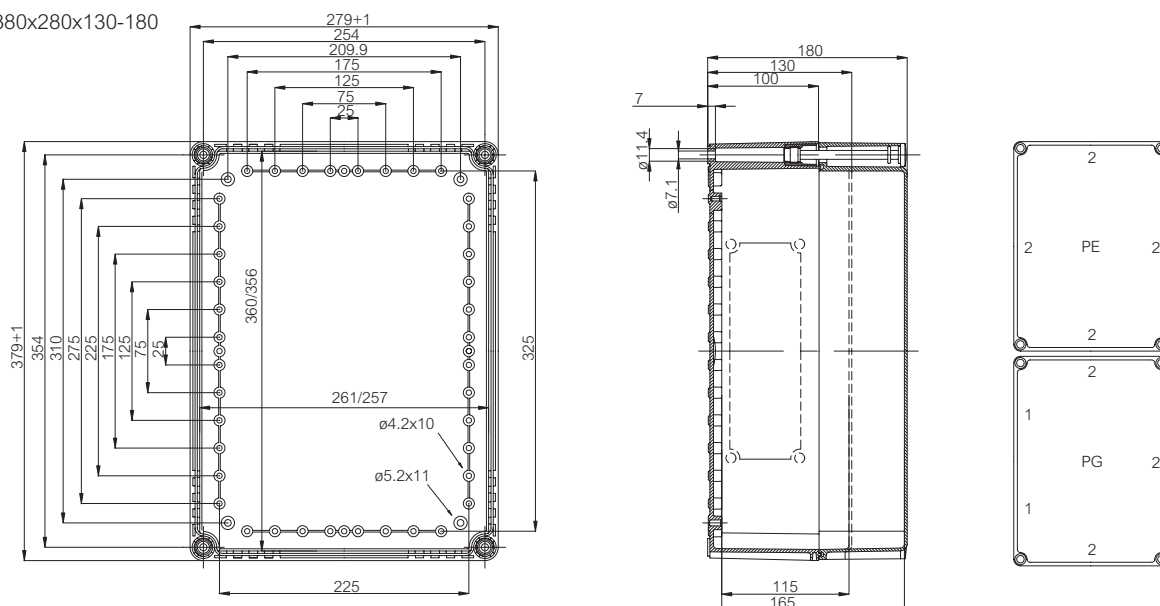
EK 380x280x130-180
