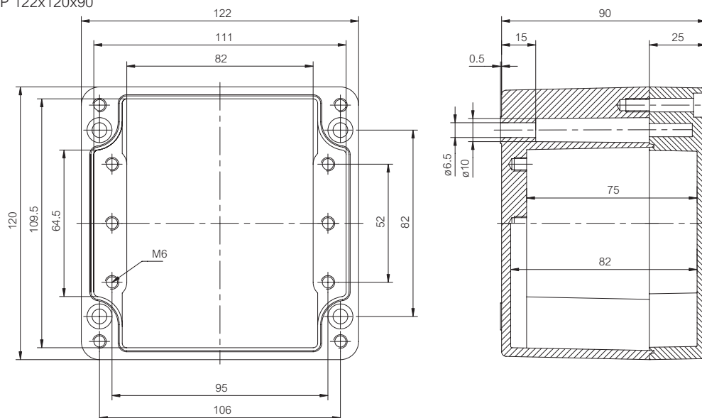
EURONORD P 122x120x90
