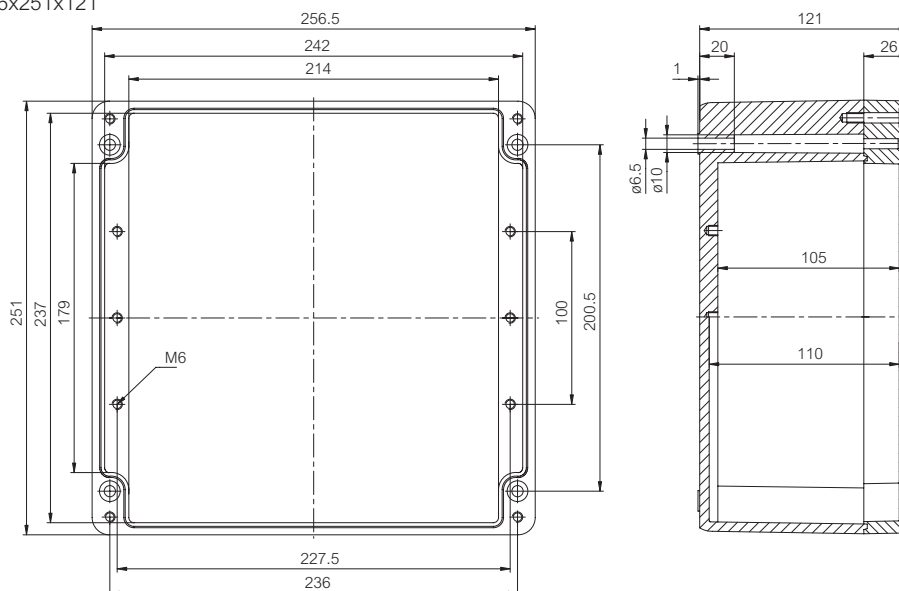
EURONORD P 256x251x121
