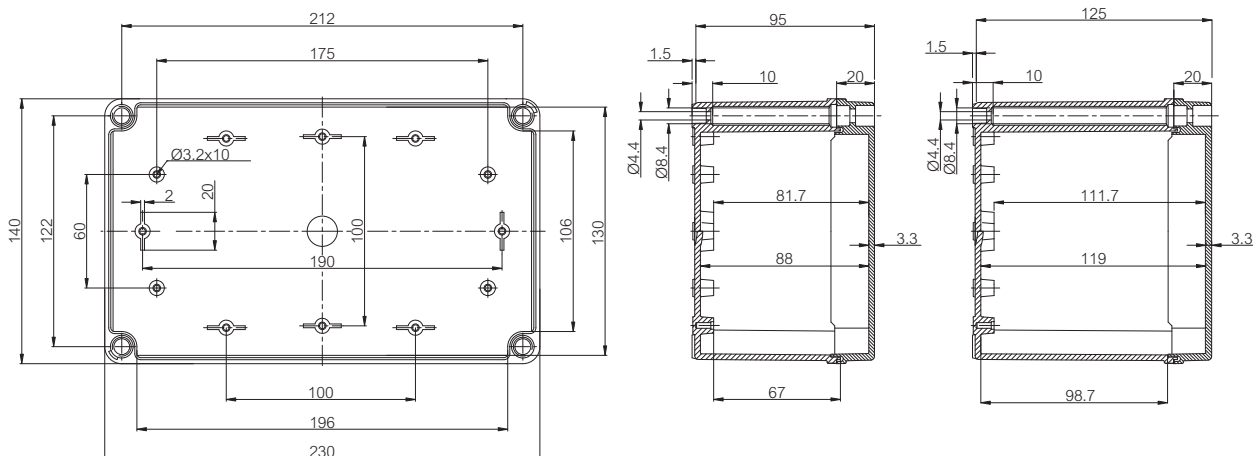
PICCOLO 230x140x95-125
