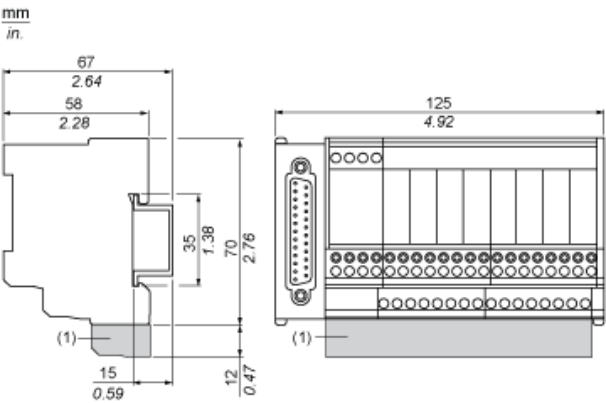
(1) ABE7BV20 / ABE7BV20E
