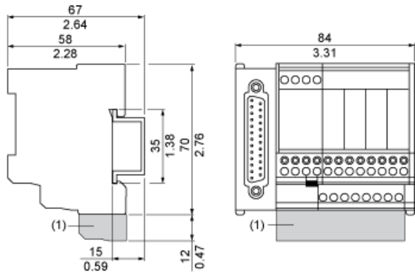
(1) ABE7BV20
