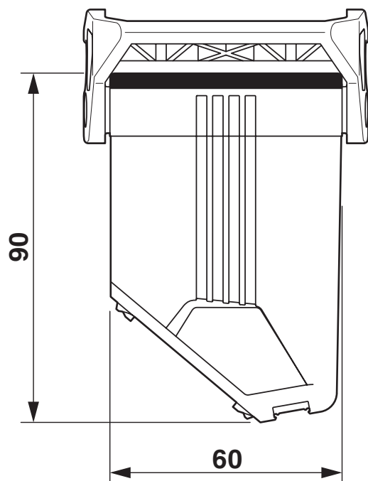
Rysunek wymiarowy
