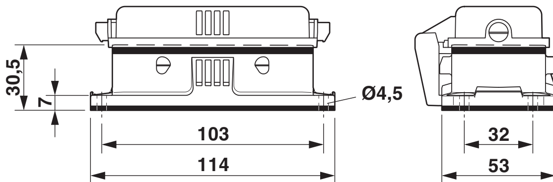
Rysunek wymiarowy
