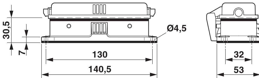
Rysunek wymiarowy
