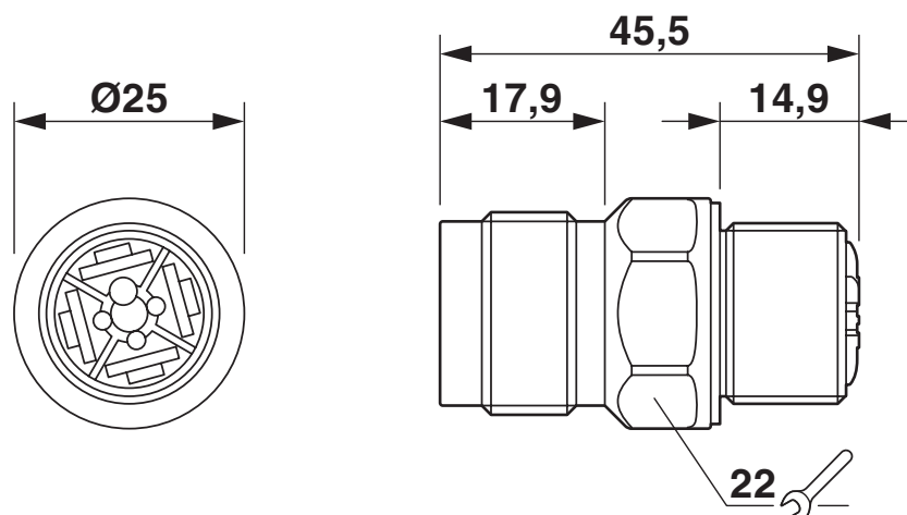
Rysunek wymiarowy
