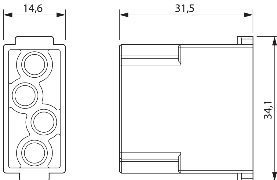
Rysunek wymiarowy
