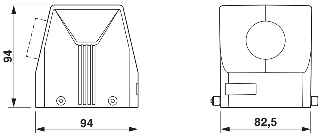
Rysunek wymiarowy
