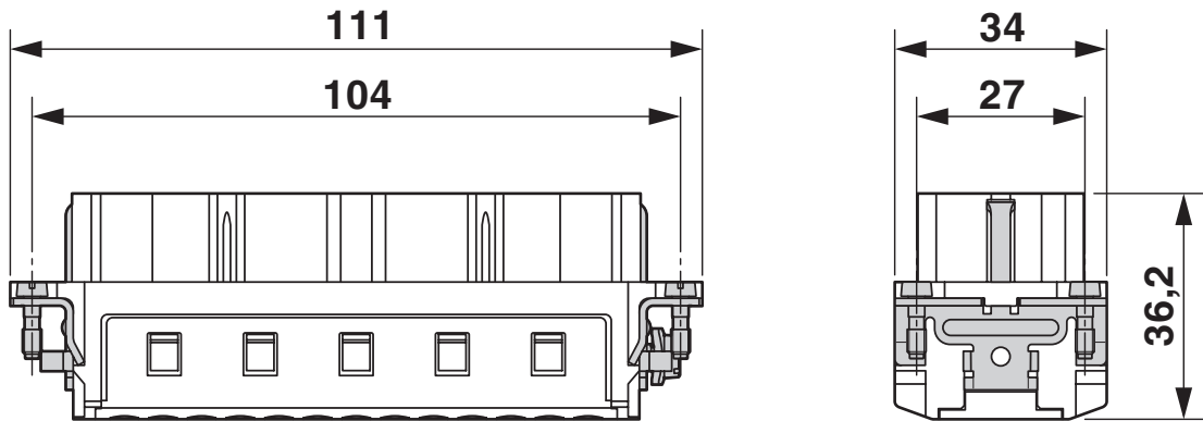
Rysunek wymiarowy
