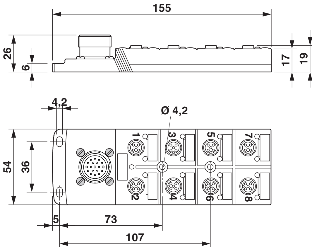
Rysunek wymiarowy
