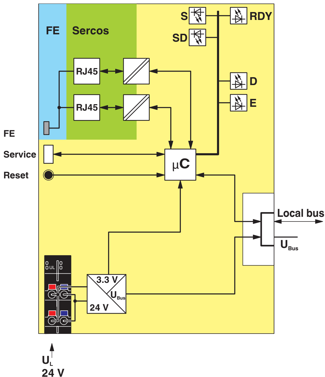
Schemat blokowy
