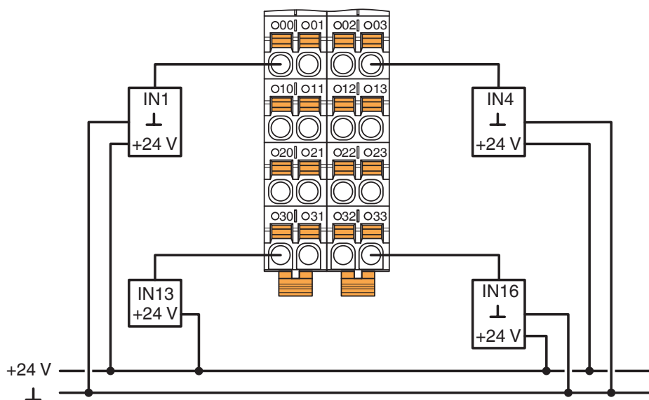
rysunek złączy
