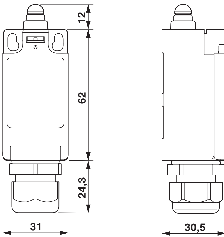
Rysunek wymiarowy
