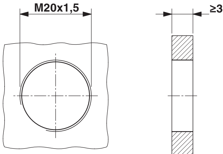
Rysunek wymiarowy
