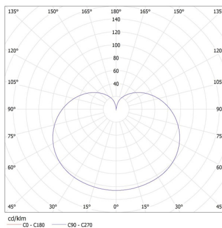
KANLUX S.A. (kat 27284) IQ-LEDDIM A60 5,5W-CW / LDC (Polar)
