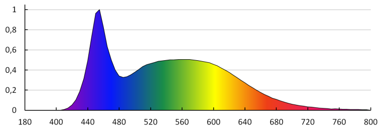
KANLUX S.A. (kat 27284) IQ-LEDDIM A60 5,5W-CW / LDC (Polar)
