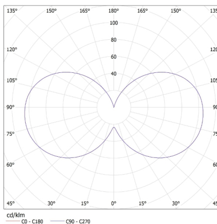
KANLUX S.A. (kat 24525) ZUBI LED 3,5W E14-WW / LDC (Polar)
