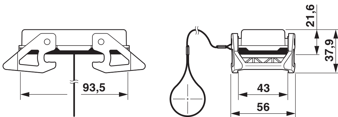
Rysunek wymiarowy
