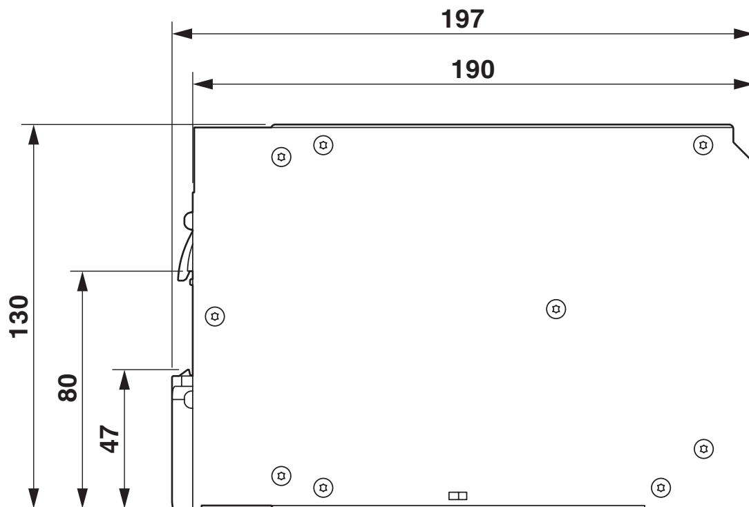
Rysunek wymiarowy
