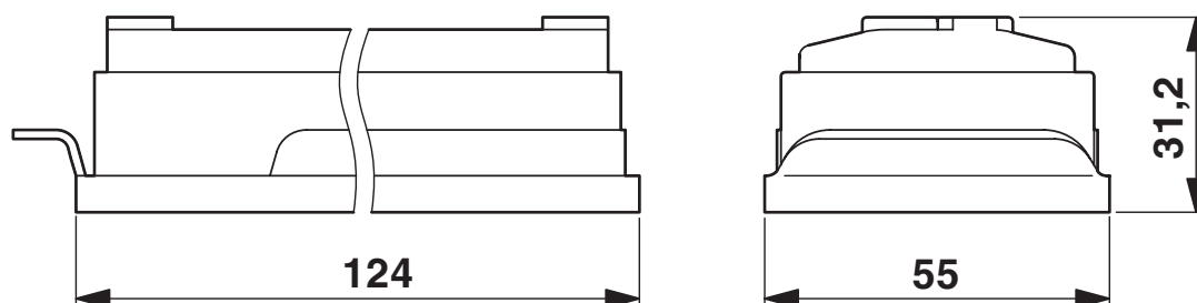
Rysunek wymiarowy
